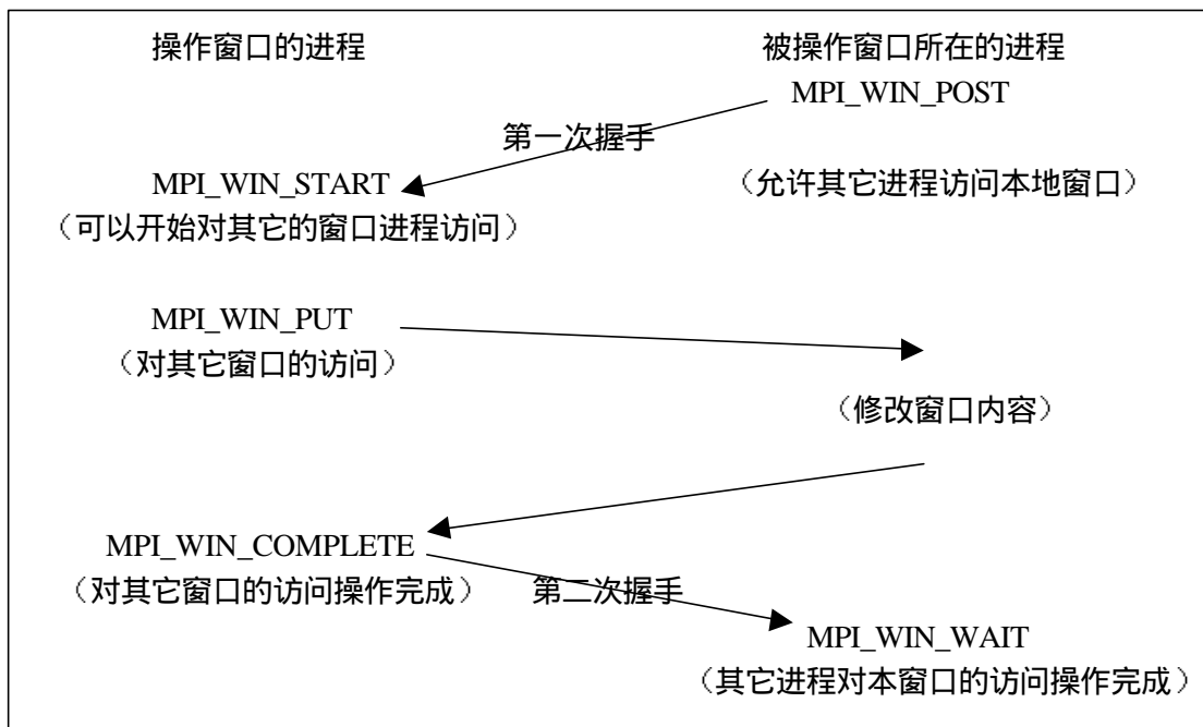
图 87 窗口握手同步方式图示
