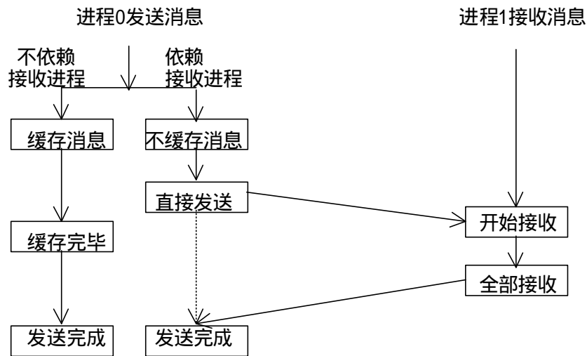
图 32 标准通信模式
