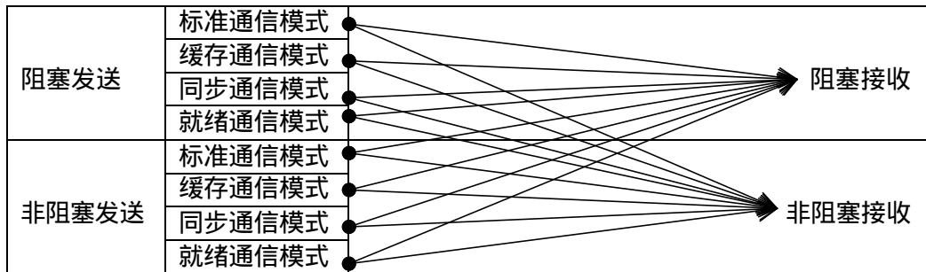
图 48 不同类型的发送与接收的匹配
