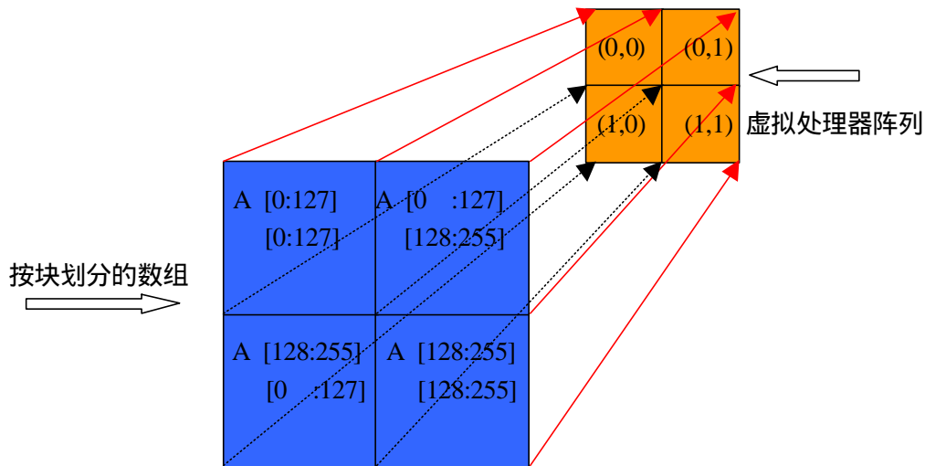
图 75 分块数组向虚拟处理器阵列的映射
