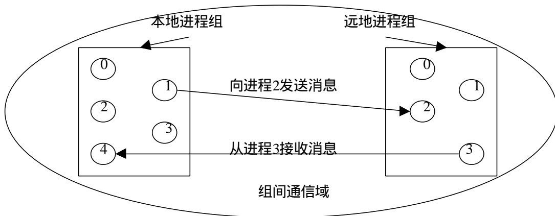
图 78 组间通信域上的点到点通信
